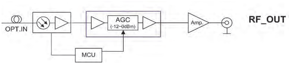
Blockschaltbild MFN-O
