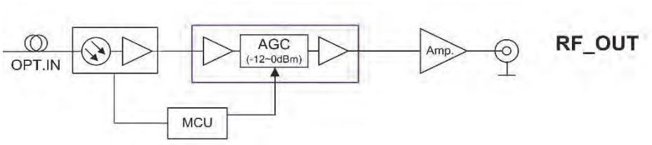
Blockschaltbild MFN-TA
