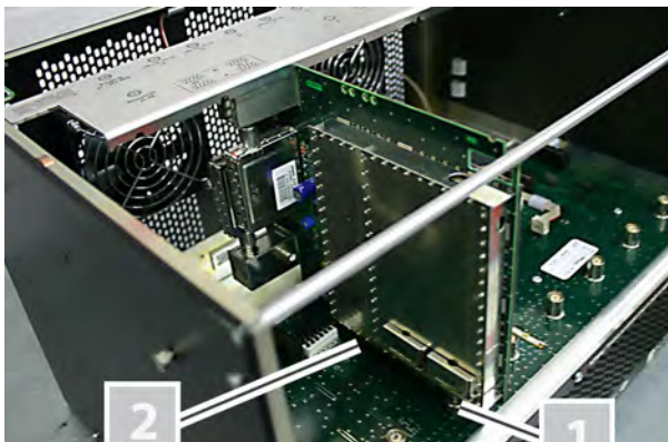
Bild 2: Einbauzustand einer Steckkarte
